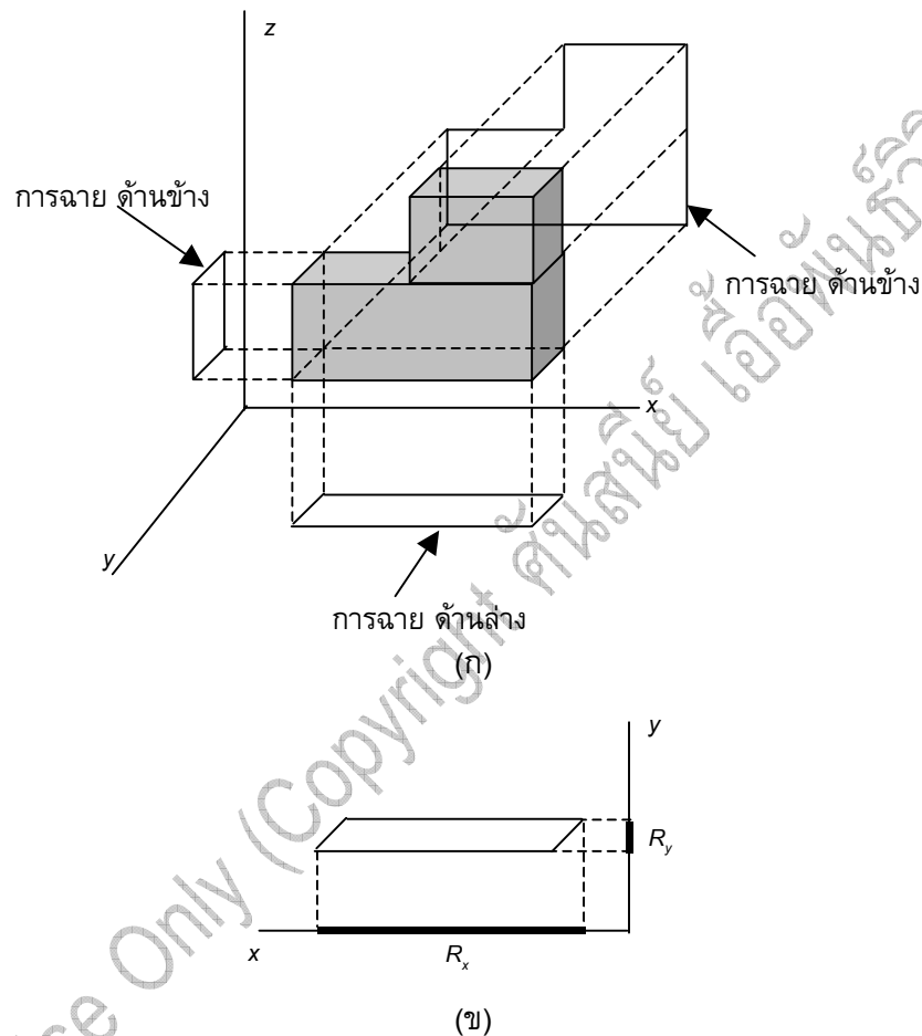
รูปที่ 4.10 (ก) การฉายความสัมพันธ์ 3 มิติไปยัง 2 มิติ (ข) การฉาย 2 มิติไปยัง 1 มิติ
