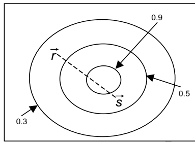
รูปที่ 3.16 แผนภาพคอนทัวร์ของ (ก) คอนเวกฟัซซีเซต (ข) ฟัซซีเซตที่ไม่คอนเวก
