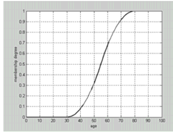
รูปที่ 1.2 membership function ของ fuzzy set ‘แก่’ (‘old’)
