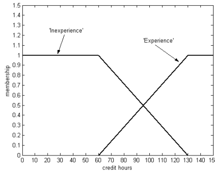
รูปที่ 3.11 ฟัซซีเซต 'Experience' และ 'Inexperience'
