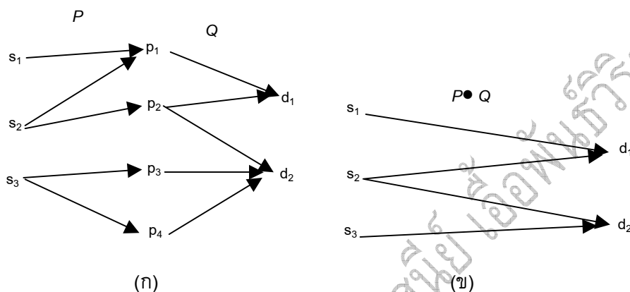
รูปที่ 4.5 (ก) ความสัมพันธ์ P และ (ข) ความสัมพันธ์ P \bullet Q
