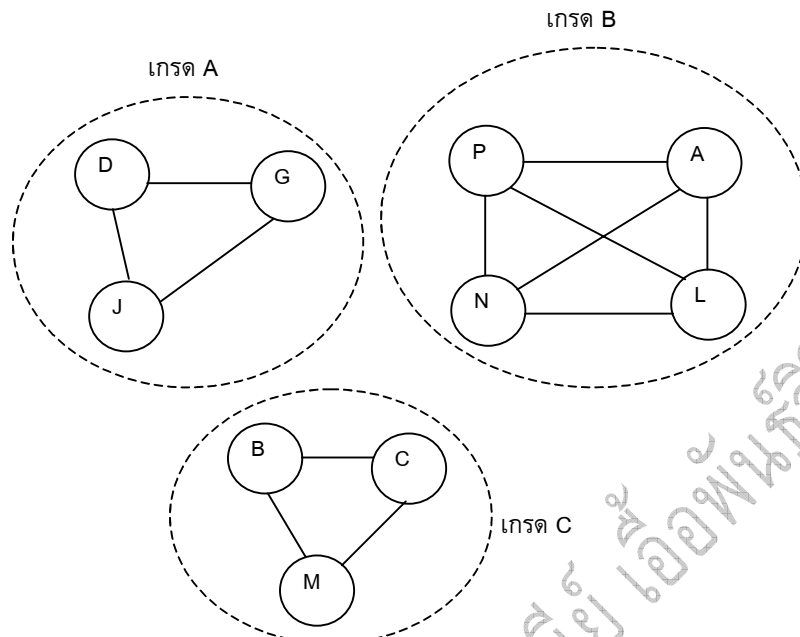
รูปที่ 4.6 ความสัมพันธ์ที่เท่ากัน (มีเกรตเท่ากัน) จากตัวอย่าง 4.1
