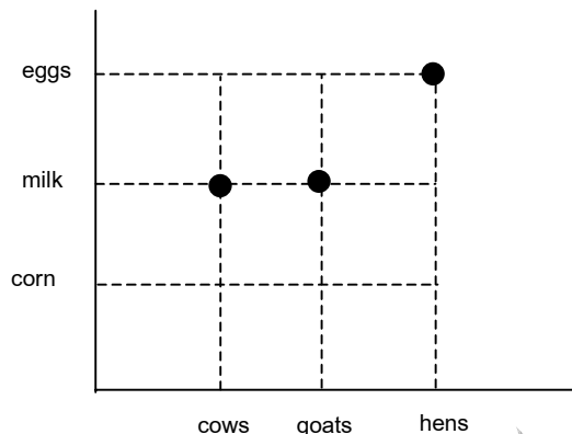
รูปที่ 4.2 ความสัมพันธ์ เป็นผลผลิตของ
