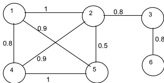
รูปที่ 5.7 ความสัมพันธ์แบบฟัซซีที่เข้ากันได้
