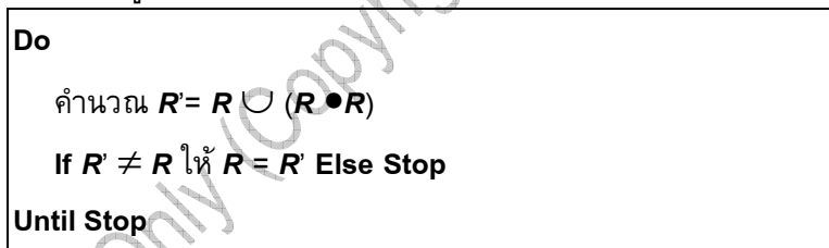
รูปที่ 5.9 อัลกอริทึมของการหา R_T
