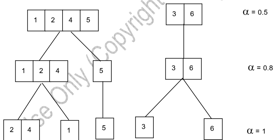
รูปที่ 5.6 ต้นไม้พาร์ติชันของ Q จากตัวอย่างที่ 5.6
