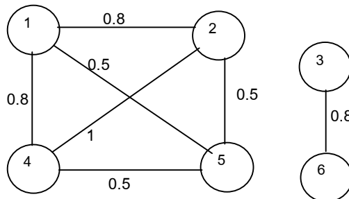
รูปที่ 5.5 ความสัมพันธ์แบบฟัซซีที่เท่ากัน Q
