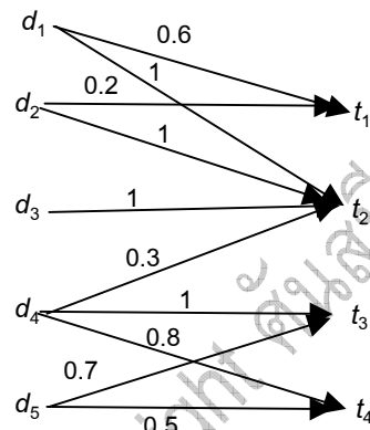
รูปที่ 5.2 การแทนแบบการส่งของความสัมพันธ์แบบฟัซซี
